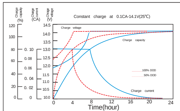
Curva de carga
